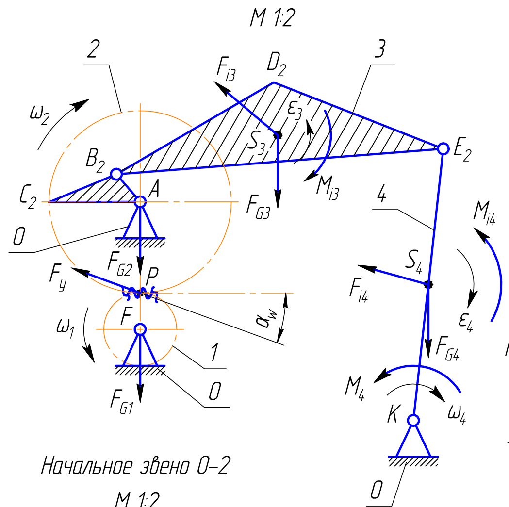
План положений механизма для положения 2
