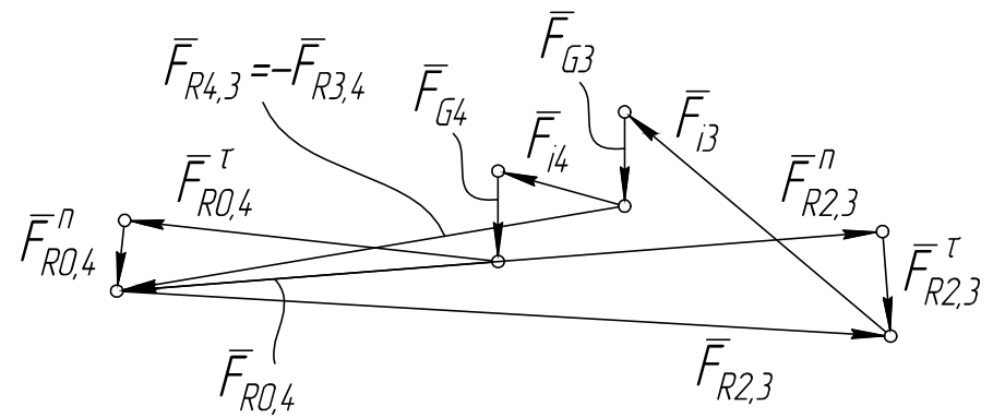
Группа Ассура 3-4 [B2,3-B3,4-B4,0]
