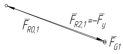
Ведущее звено 0-1
