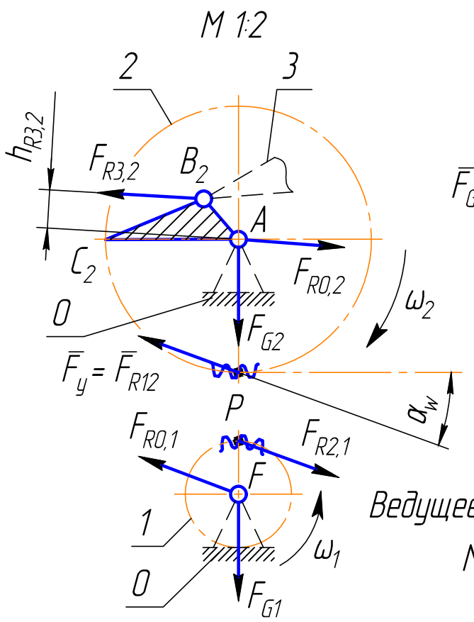
Начальное звено 0-2
