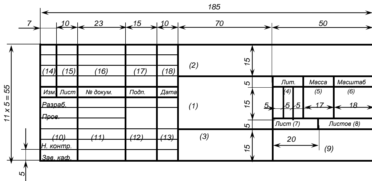
Рисунок С.1 – Основная надпись для чертежей и схем (первый лист) по ГОСТ 2.104, форма 1
