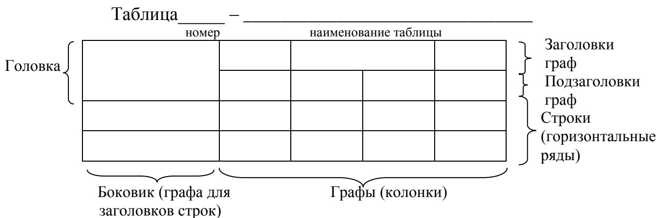
Рисунок 1 – Структура таблицы
