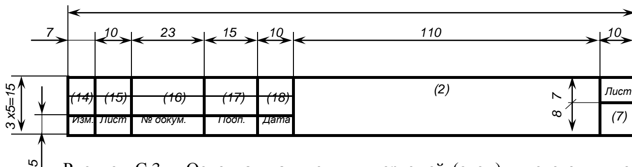
Рисунок С.3 – Основная надпись для чертежей (схем) и текстовых конструкторских документов (последующие листы) по ГОСТ 2.104, форма 2а 185
