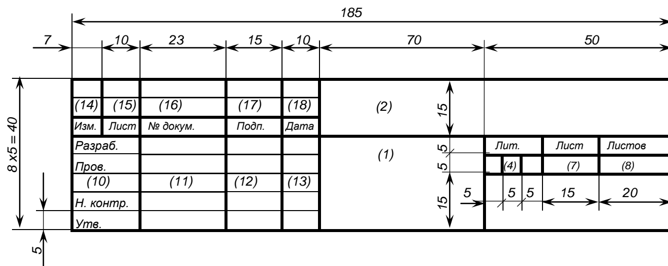
Рисунок С.2 – Основная надпись для текстовых конструкторских документов (первый лист) по ГОСТ 2.104, форма 2
