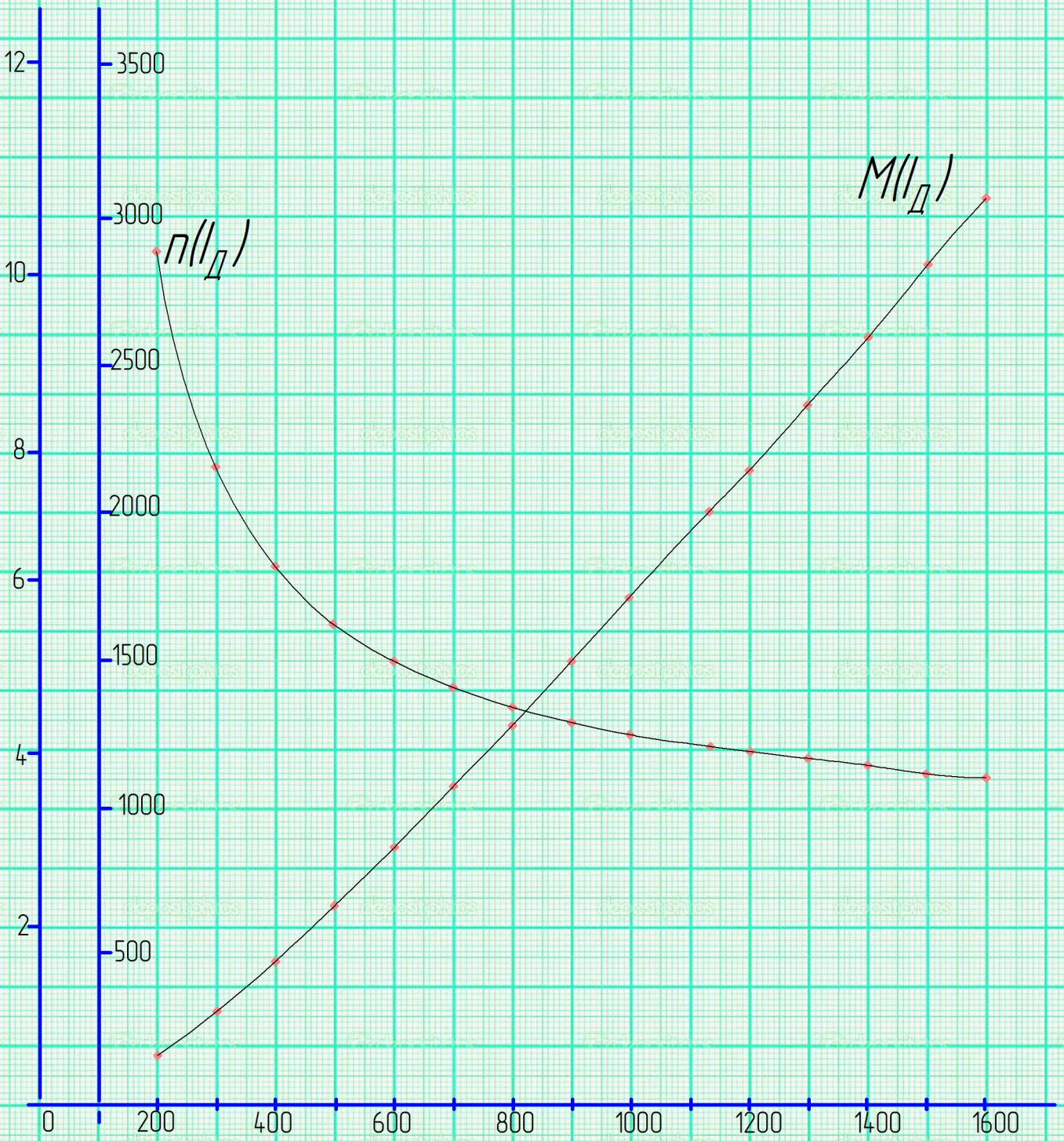
Рисунок 1. Электромеханические характеристики тягового двигателя AL-44P
