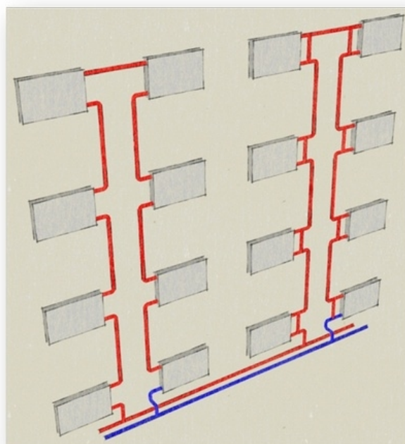
Рисунок 1 – Однотрубная система отопления с нижней подачей
