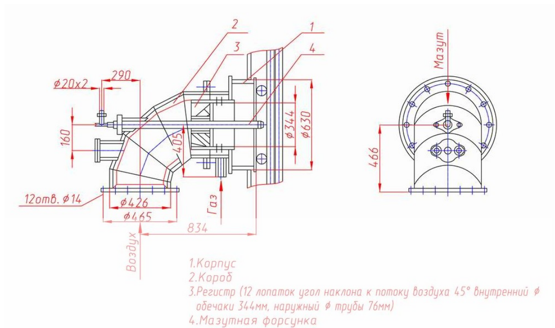
Рис. 5 – Горелка газомазутная МГМГ
