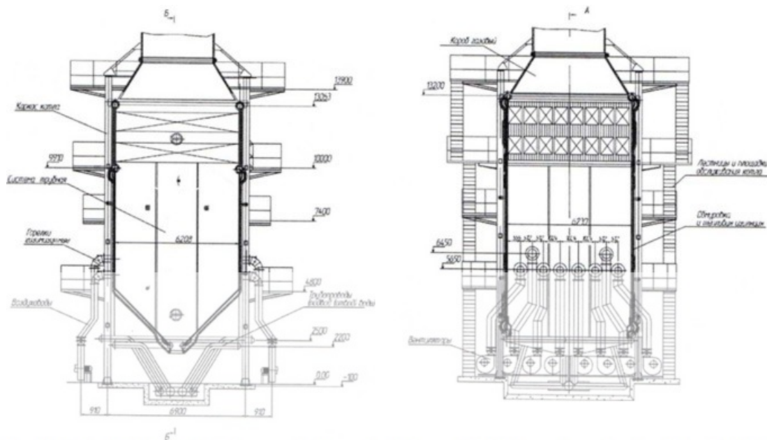
Рис. 3 – Пиковый теплофикационный водогрейный котел типа ПТВМ-100
